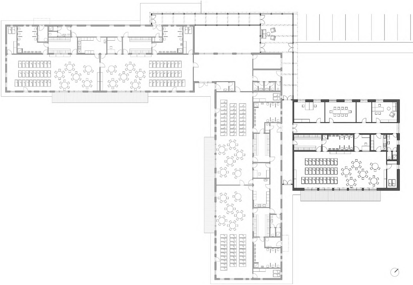
půdorys přízemí 1:200
